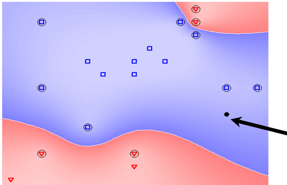
شکل (5-22): پیش گوئی توسط c = \inf , erbf
