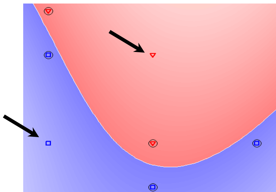
شکل ( 4-14 ) : نقش یکتای SV ها در عمل جداسازی
