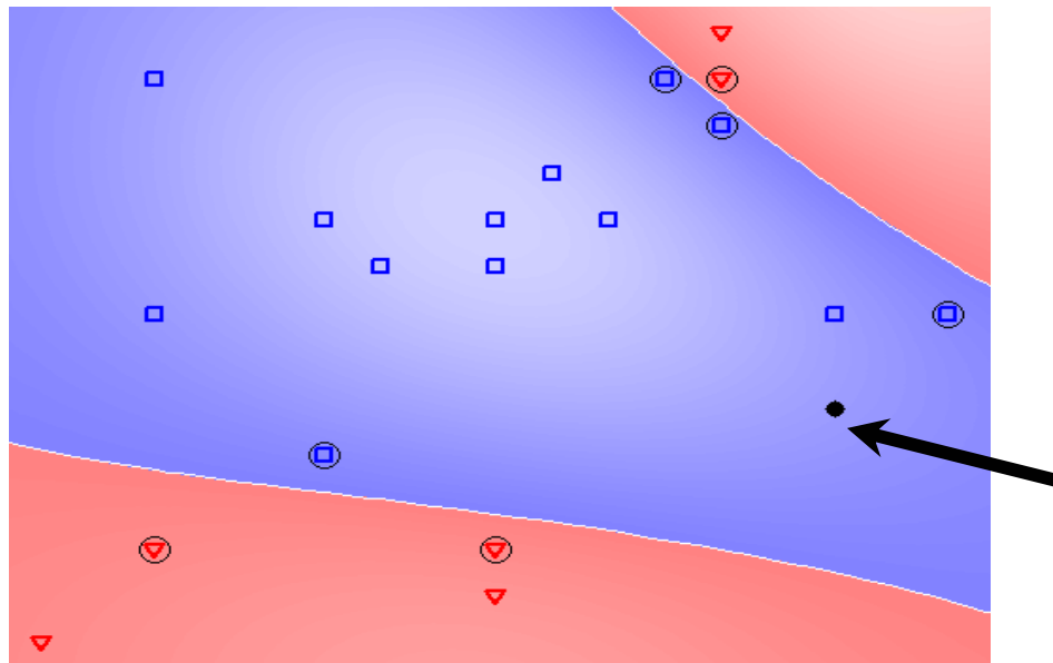
شکل (5-23): پیش گوئی توسط c = \inf , rbf
