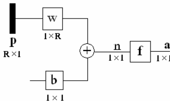
شکل ( 2-5 ) : فرم ساده شده نرون با چند ورودی
