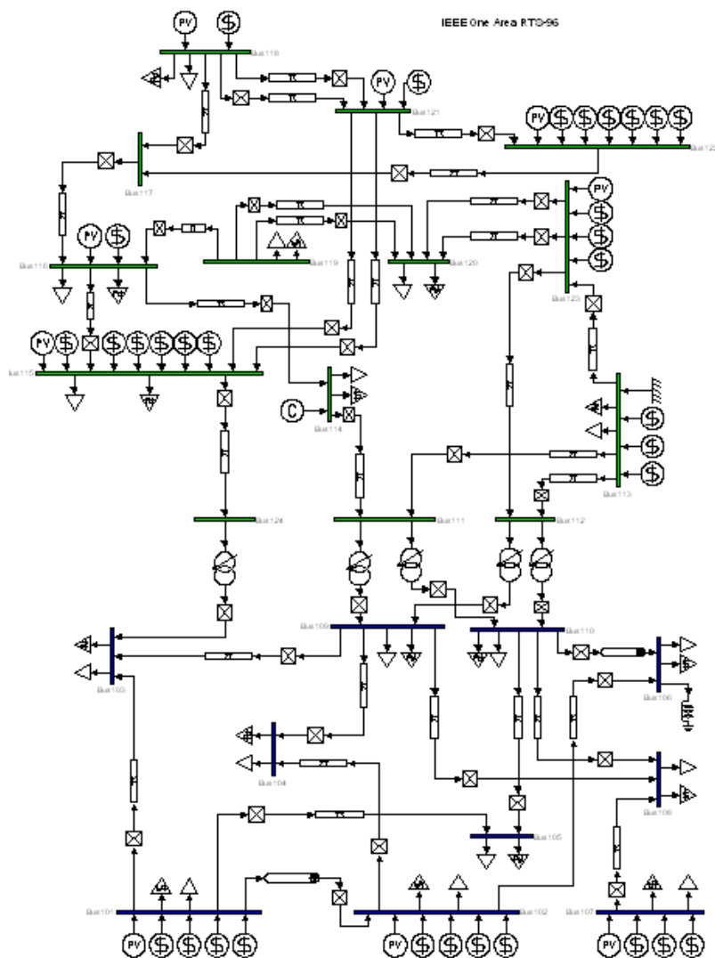
شکل ( 24-5) : شبکه 24 باس باره استاندارد
