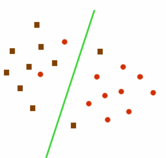
شکل (3-7) : داده‌های تفکیک نا پذیر خطی
