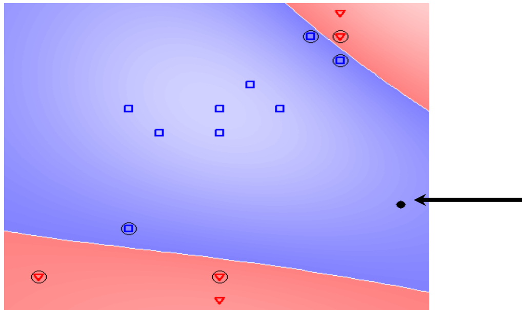
شکل (5-18): پیش گوئی در مورد یک نقطه c = \inf , r_b f
